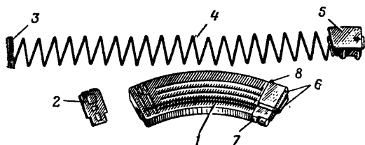
Рис. 39. Магазин:
