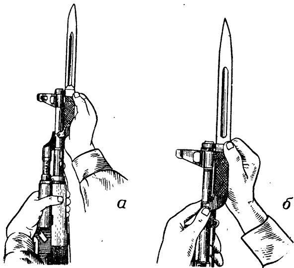
Рис. 26. Снятие штыка:
