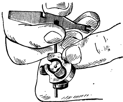
Рис. 14. Выталкивание шпильки при разборке затвора
