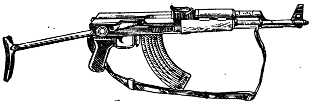
Рис. 1. Общий вид автомата Калашникова (АК): а — с деревянным прикладом; б — с металлическим прикладом
