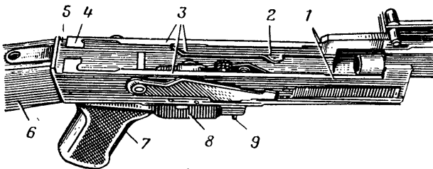
Рис. 28. Ствольная коробка:
