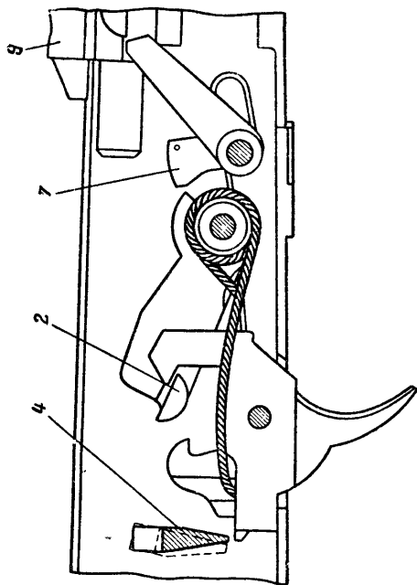
Рис. 45. Положение частей ударно-спускового механизма перед выстрелом: 2 — курок; 4 — сектор переводчика; 7 — выступ автоспуска; 9 — защелка
